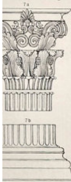
Basis vom Monument des Lysikrates zu Athen.
